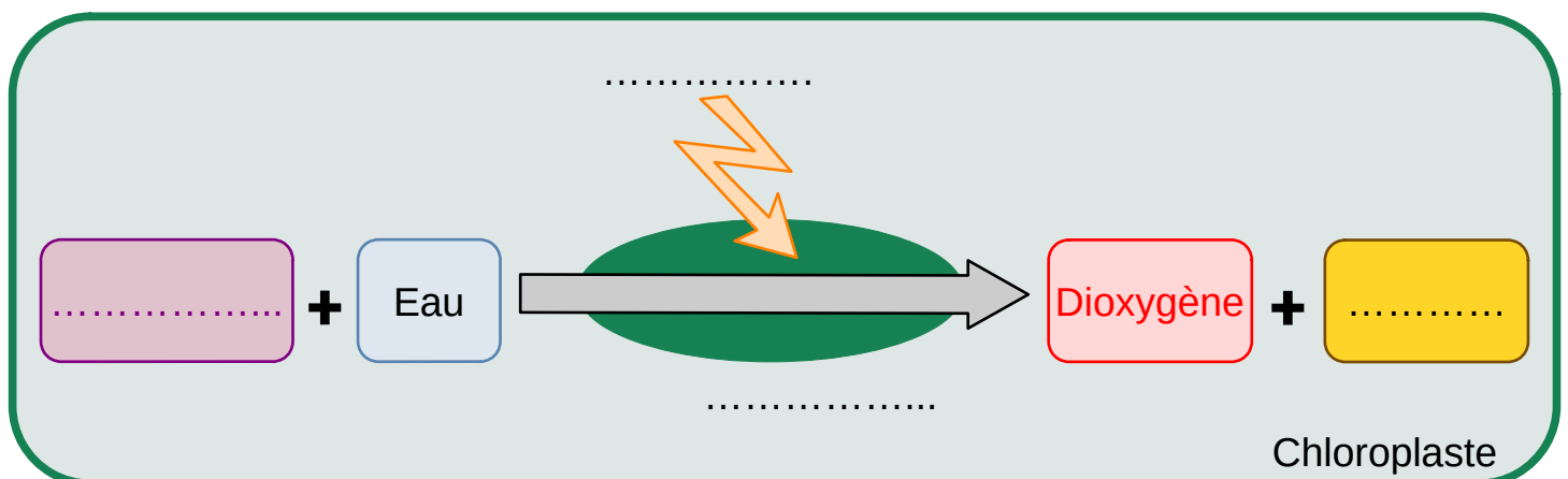
Schéma de l'équation de la photosynthèse
